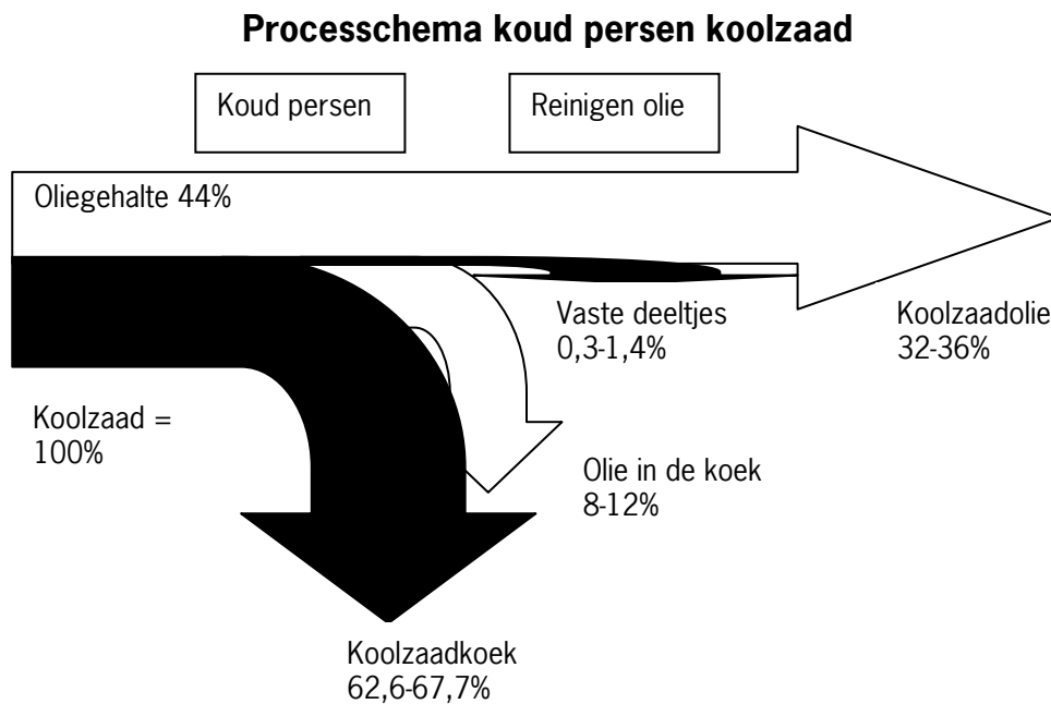
Figuur 1: Stromen uit persing van koolzaad (Fenchau, 2005)
